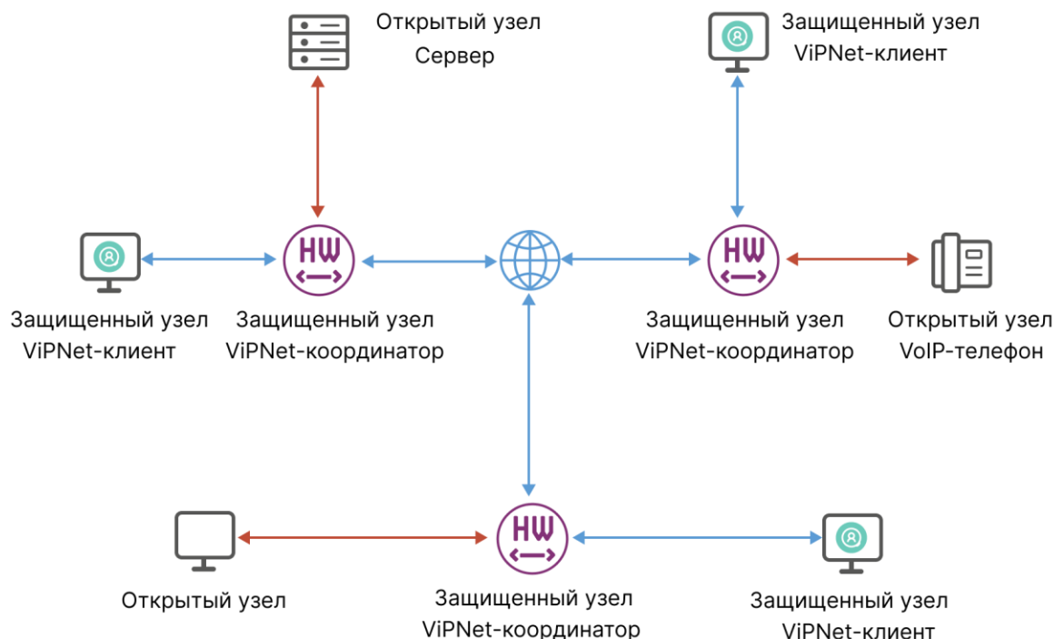
Рисунок 1. Типы узлов сети ViPNet
