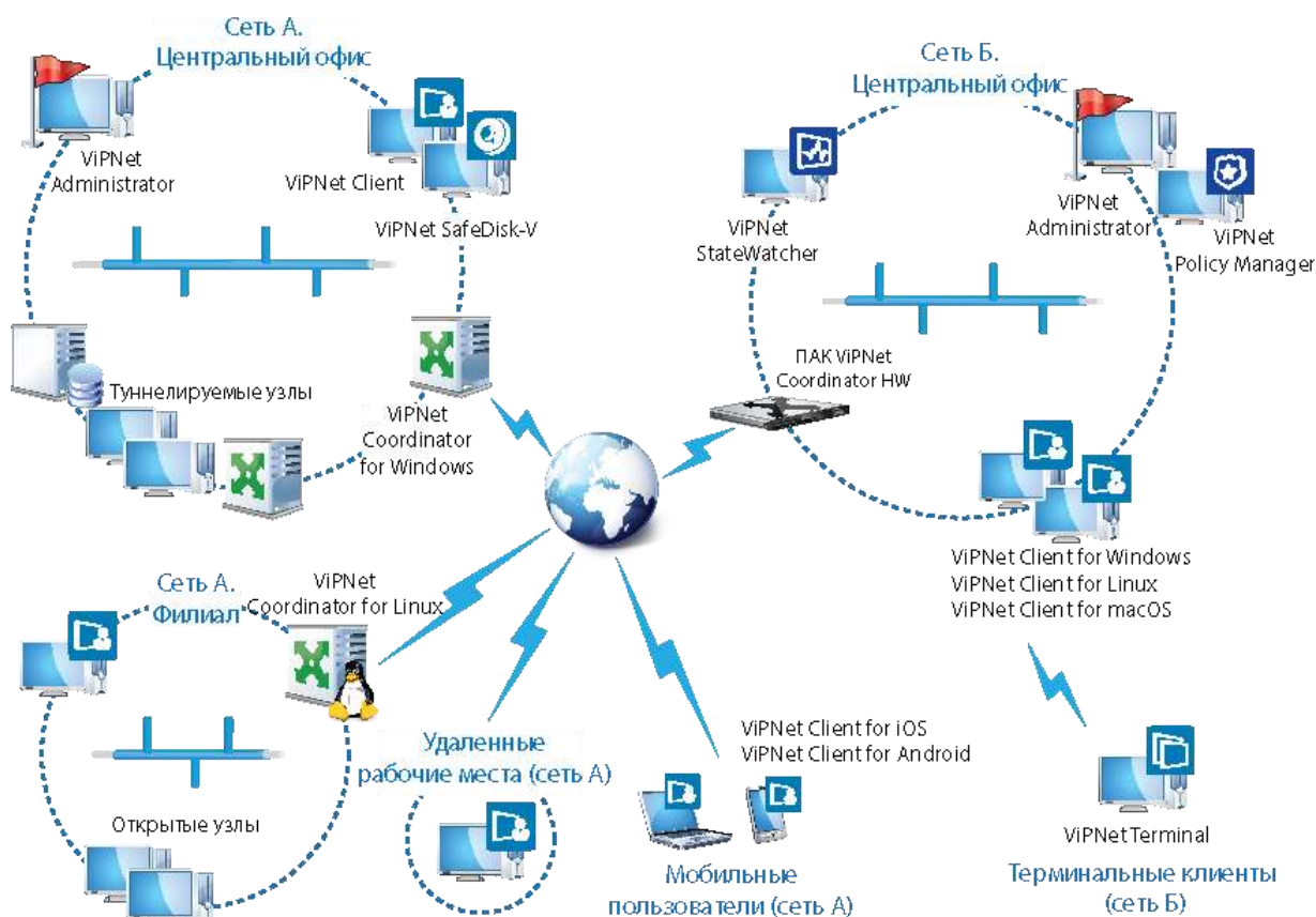
Рисунок 1. Схема сети ViPNet под управлением ПО ViPNet Administrator
