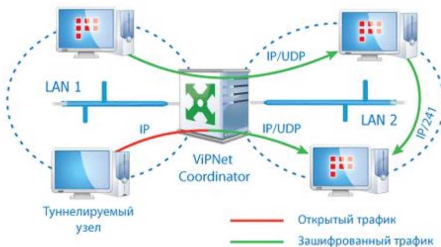
Рисунок 9. Координатор осуществляет туннелирование и трансляцию адресов для ViPNet-соединений
