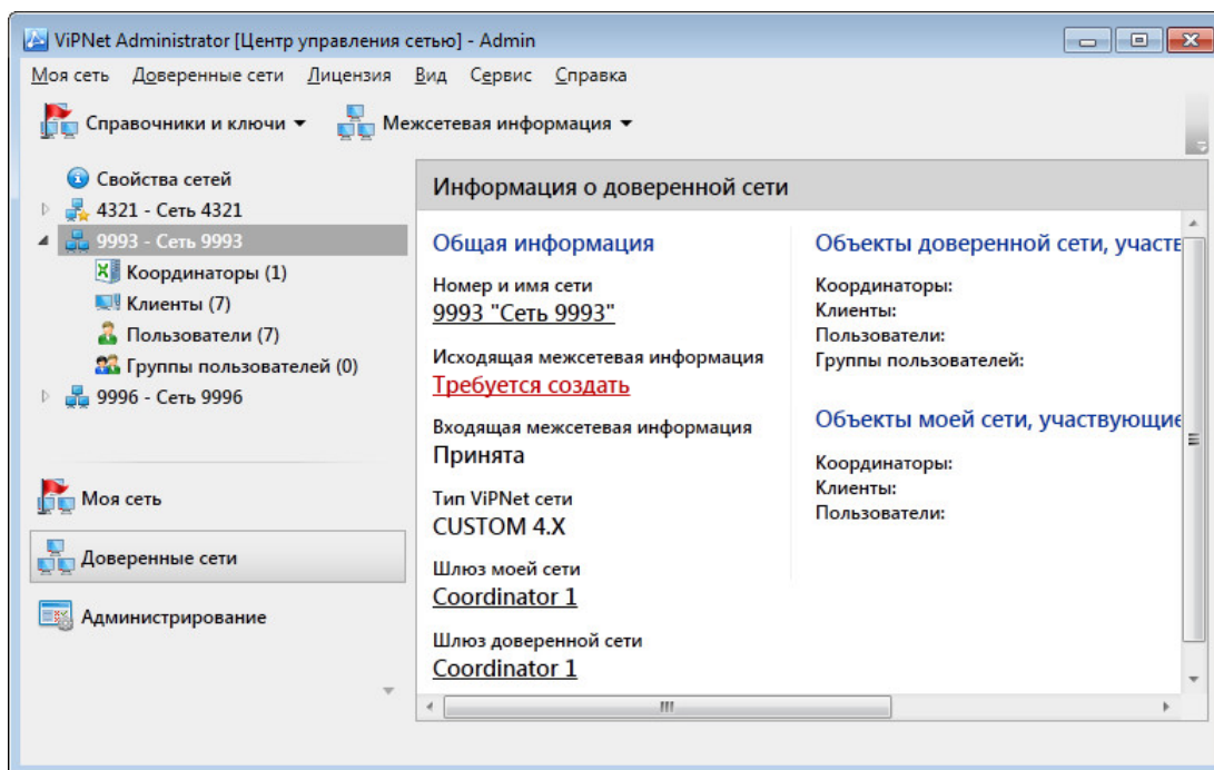
Рисунок 22. Доверенная сеть
