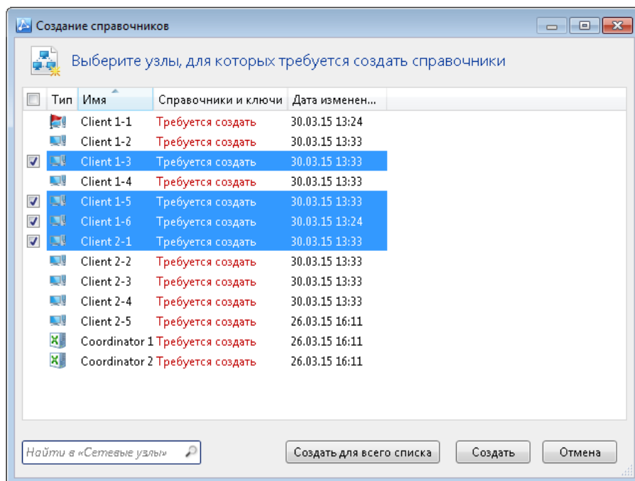
Рисунок 39. Создание справочников
