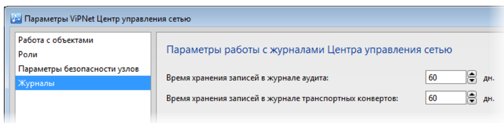
Рисунок 34. Параметры журналов
