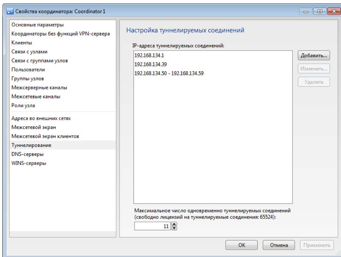
Рисунок 57. Настройка туннелирования
