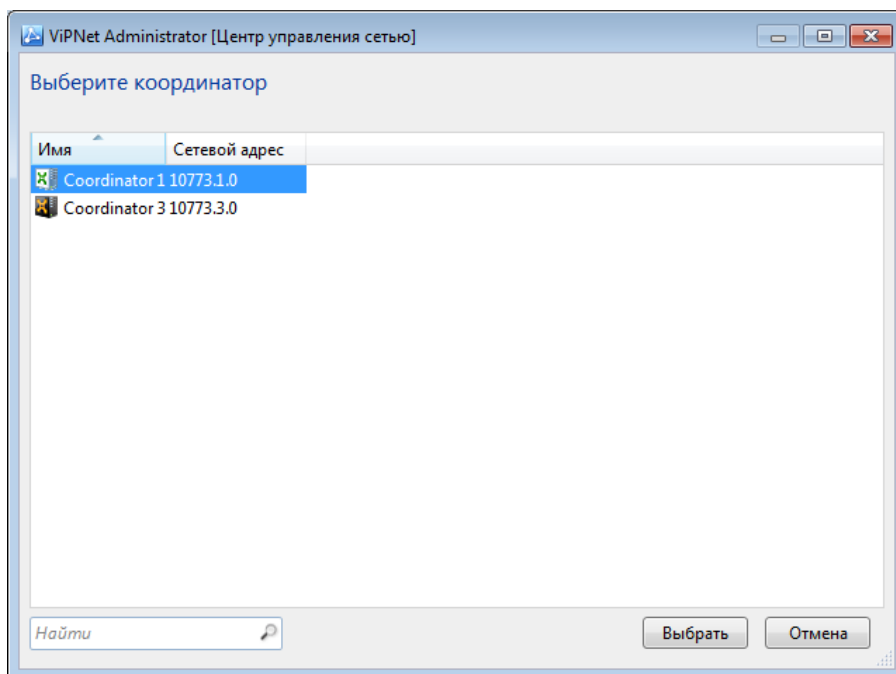
Рисунок 59. Выбор координатора
