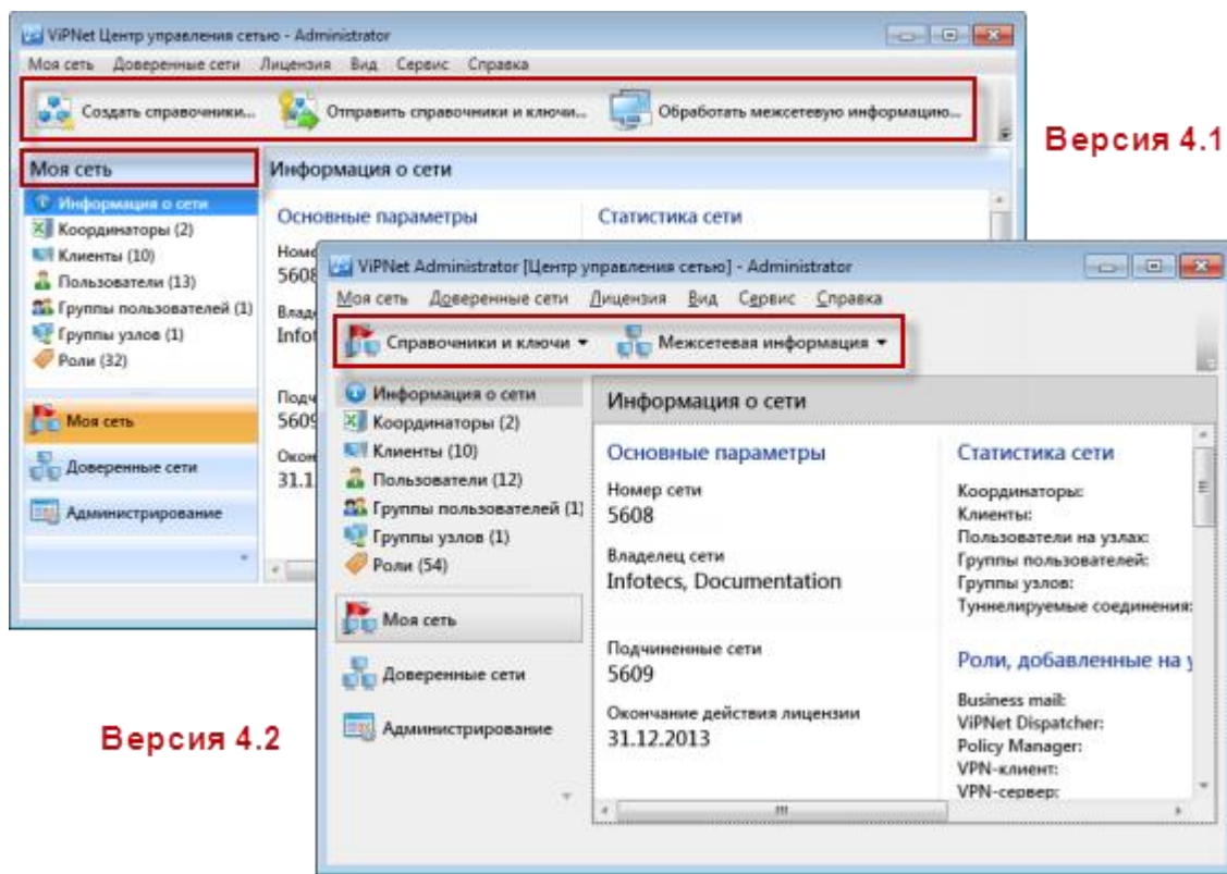
Рисунок 167. Оптимизированный интерфейс
