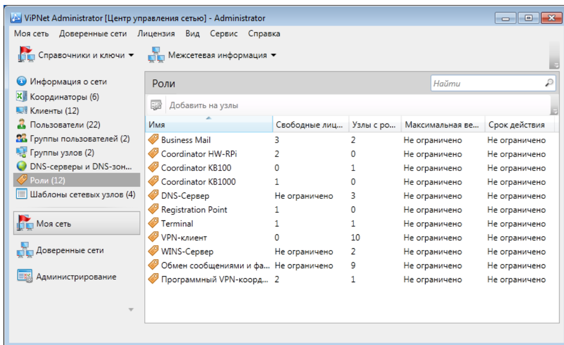
Рисунок 69. Список ролей
