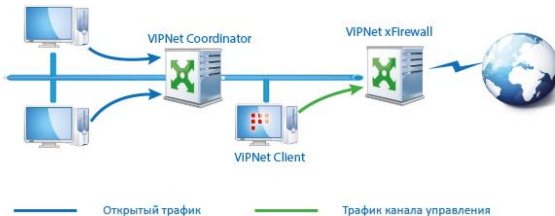
Рисунок 7. Расположение ViPNet Client и ViPNet xFirewall в одной подсети
